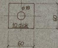
85 Isolierscheibe 10 x 60 x 60
