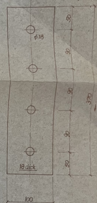
83 Isolierklotz 18 x 100 x 370
