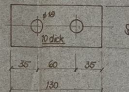
84 Isolierscheibe 10 x 60 x 130
