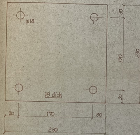
81 Isolierklotz 18 x 230 x 230
