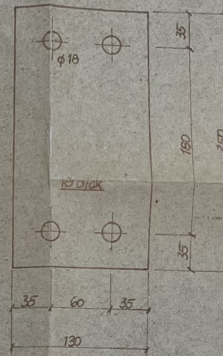
82 Isolierklotz 18 x 130 x 250
